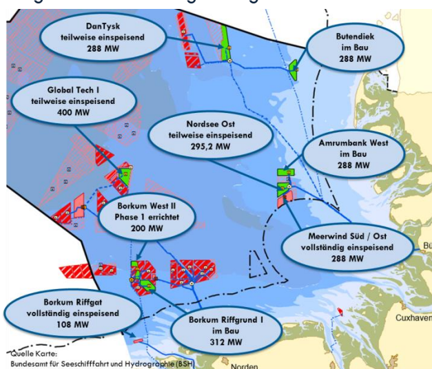
Abbildung 4: Im Jahr 2014 im Bau befindliche, errichtete und neu einspeisende OWP in der Nordsee
