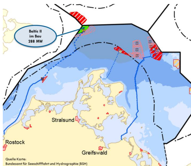
Abbildung 5: Im Jahr 2014 im Bau befindlicher OWP in der Ostsee
