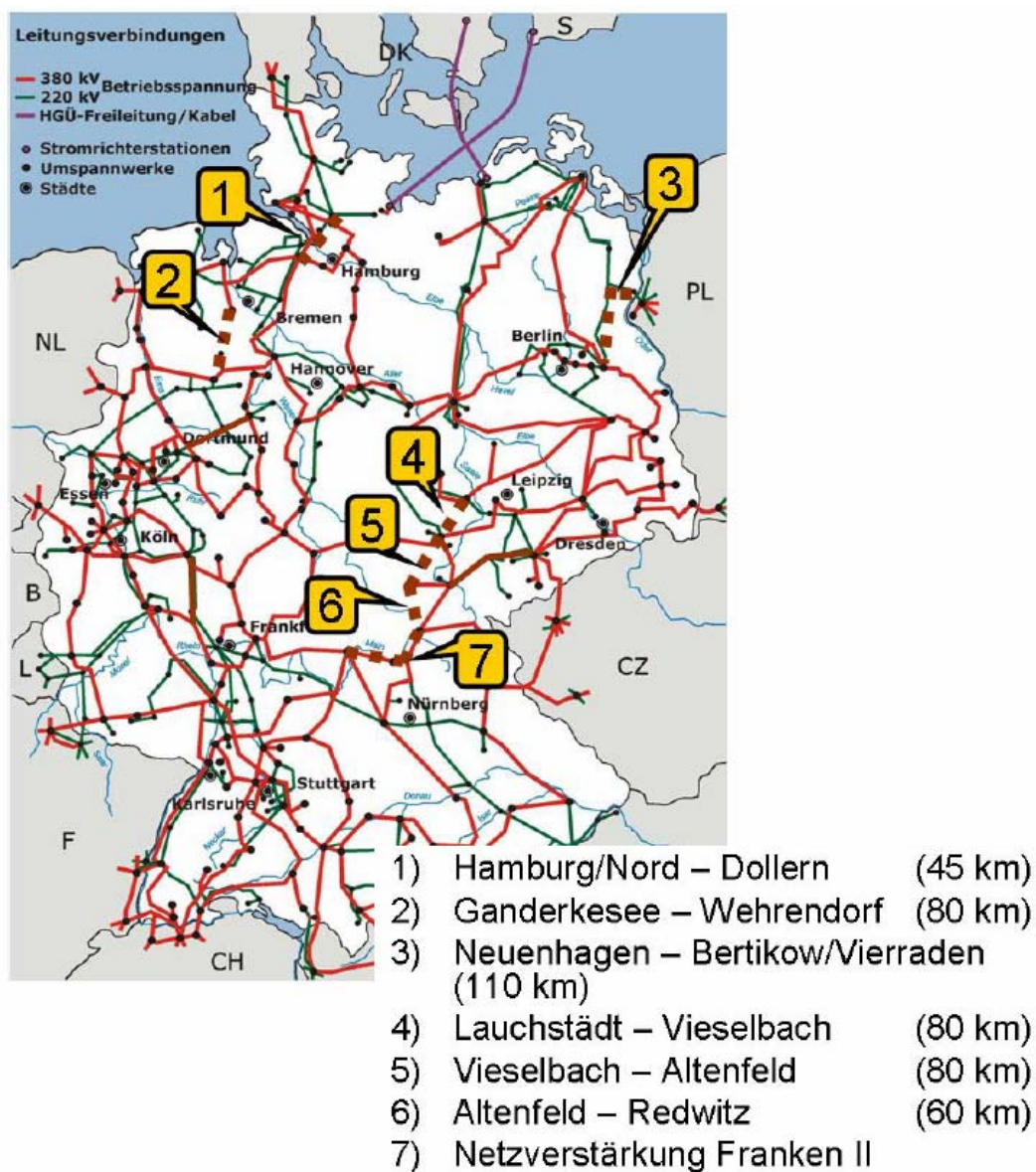
Abbildung 2: Netzverstärkungen und Netzausbau im Höchstspannungsübertragungsnetz zwischen 2007 und 2010
