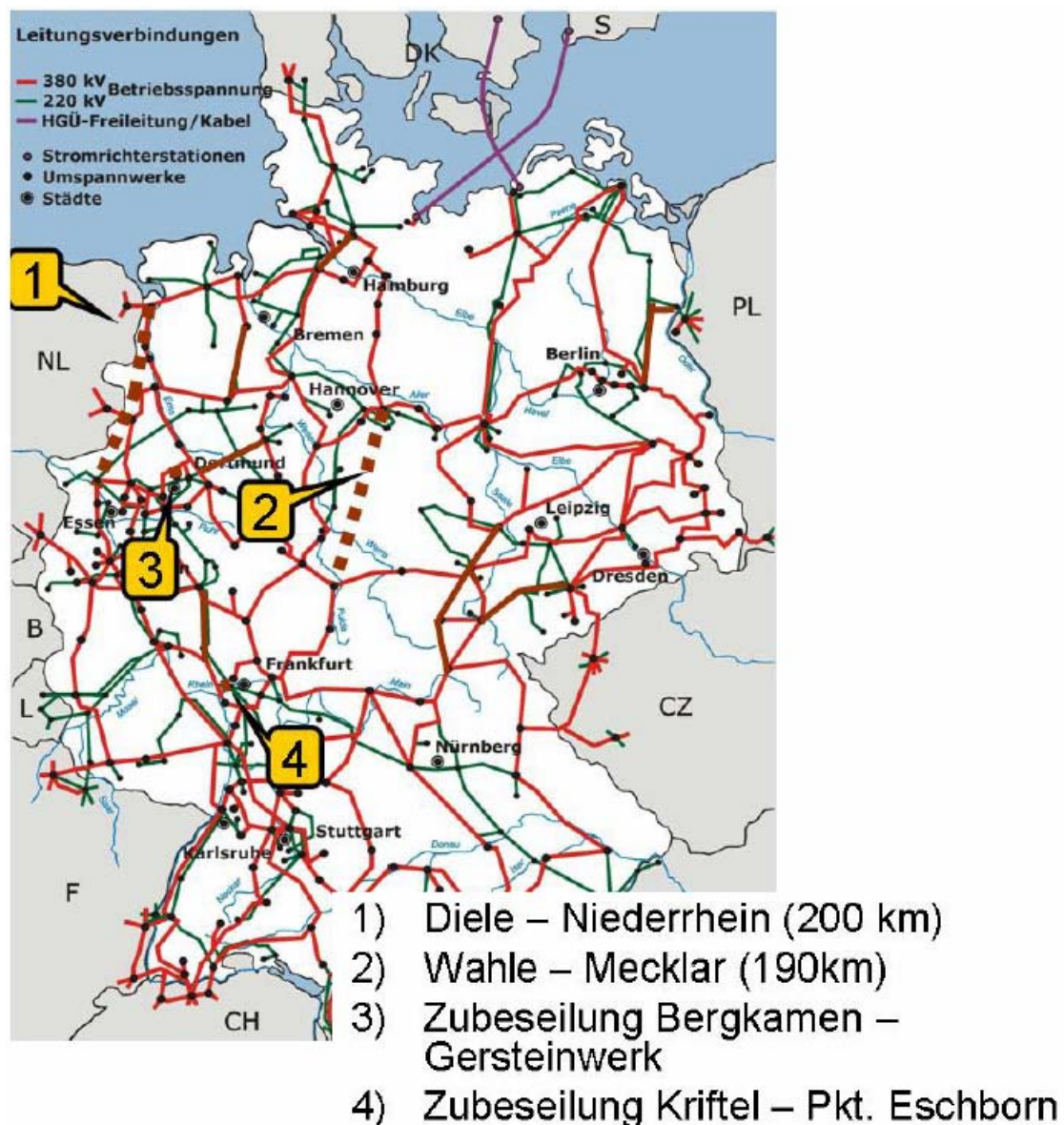
Abbildung 3: Netzverstärkungen und Netzausbau zwischen 2010 und 2015
